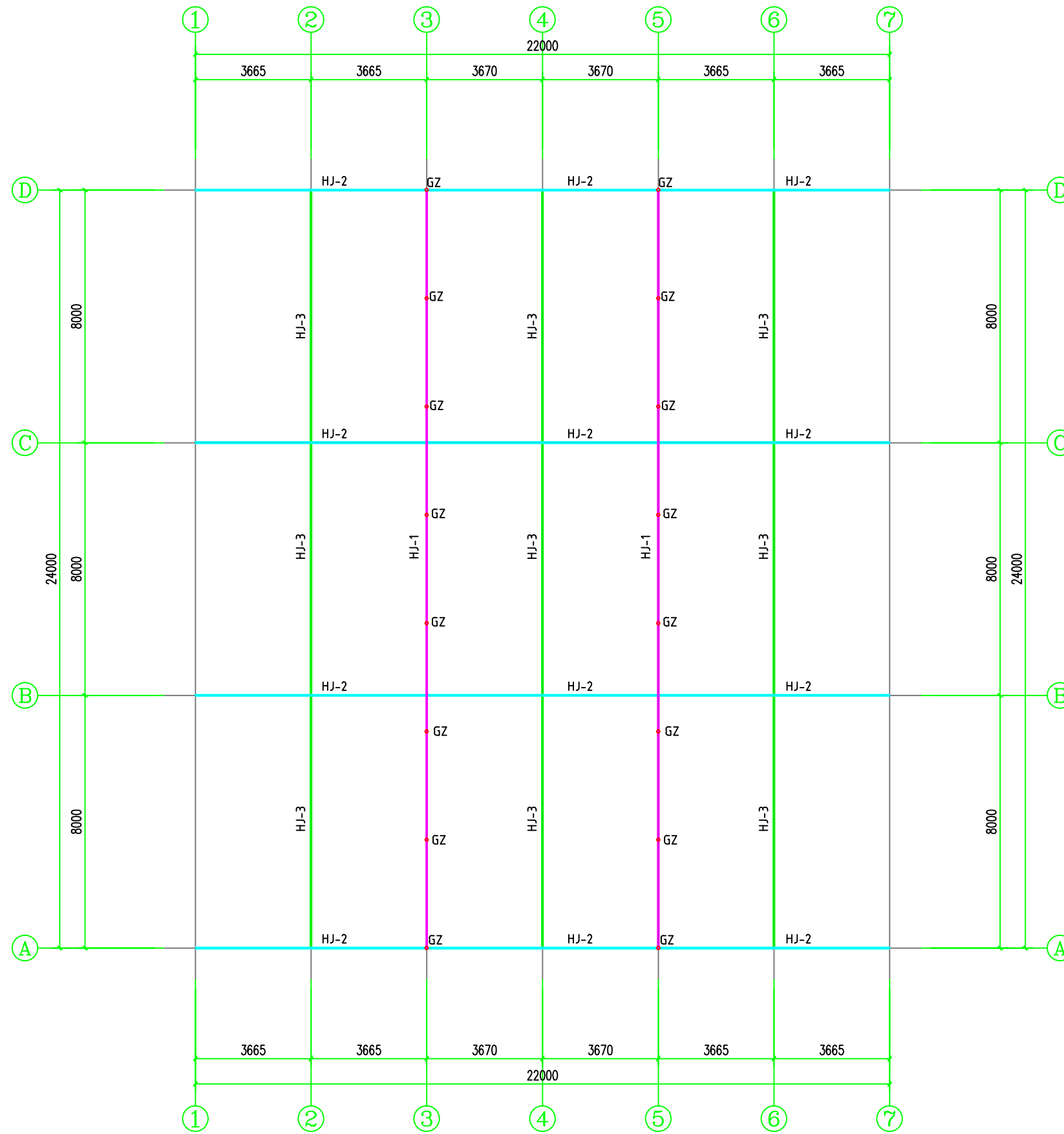
屋架平面布置图
