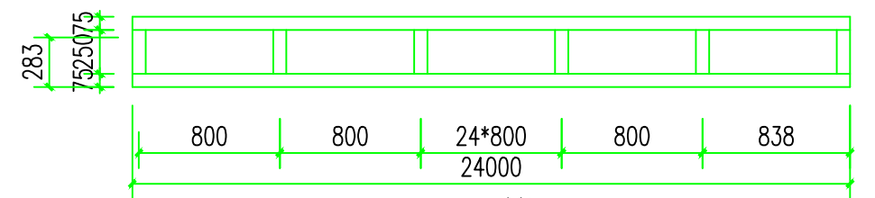
HJ-3大样图
