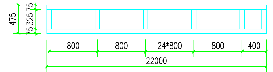
HJ-2大样图
