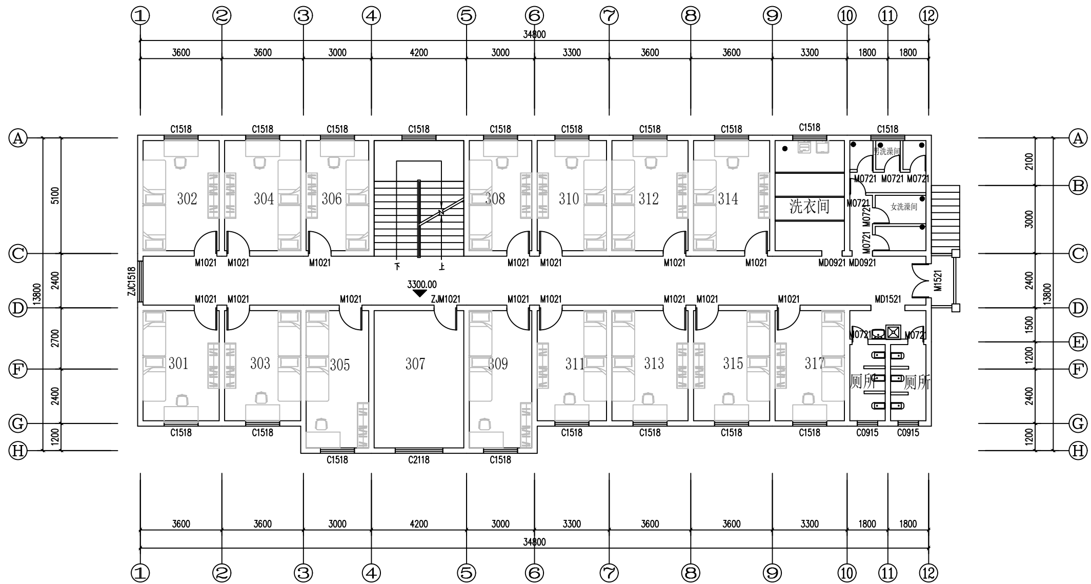
三层改造平面图
